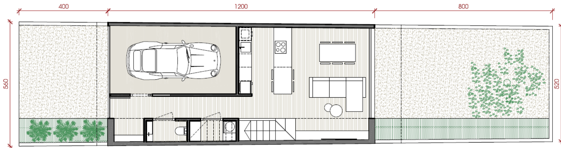
PLANTA BAIXA
